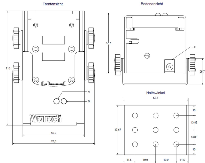
Schemazeichnung WTC680
