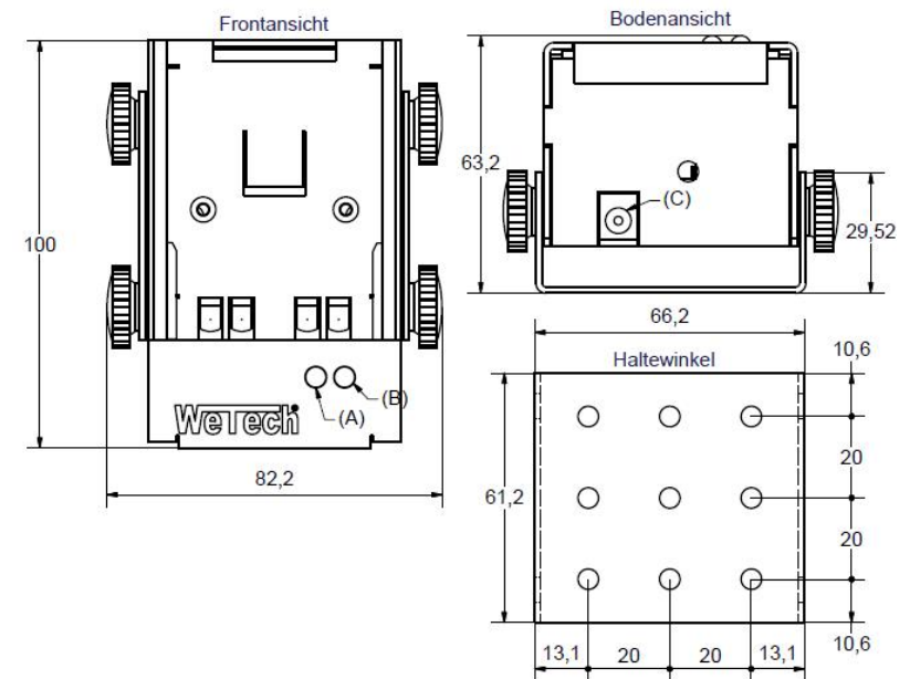
Schemazeichnung WTC1704
